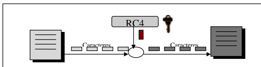
Figura 6.4.1: RC4.
