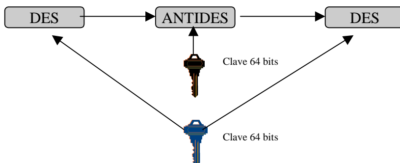
Figura 6.2.1: Triple DES.
